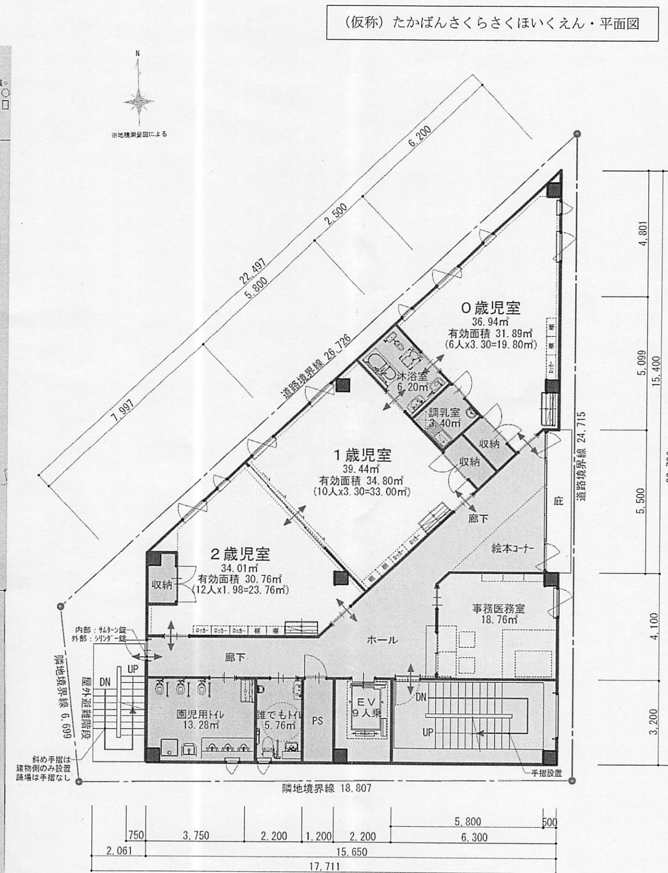
〔2階平面図〕
