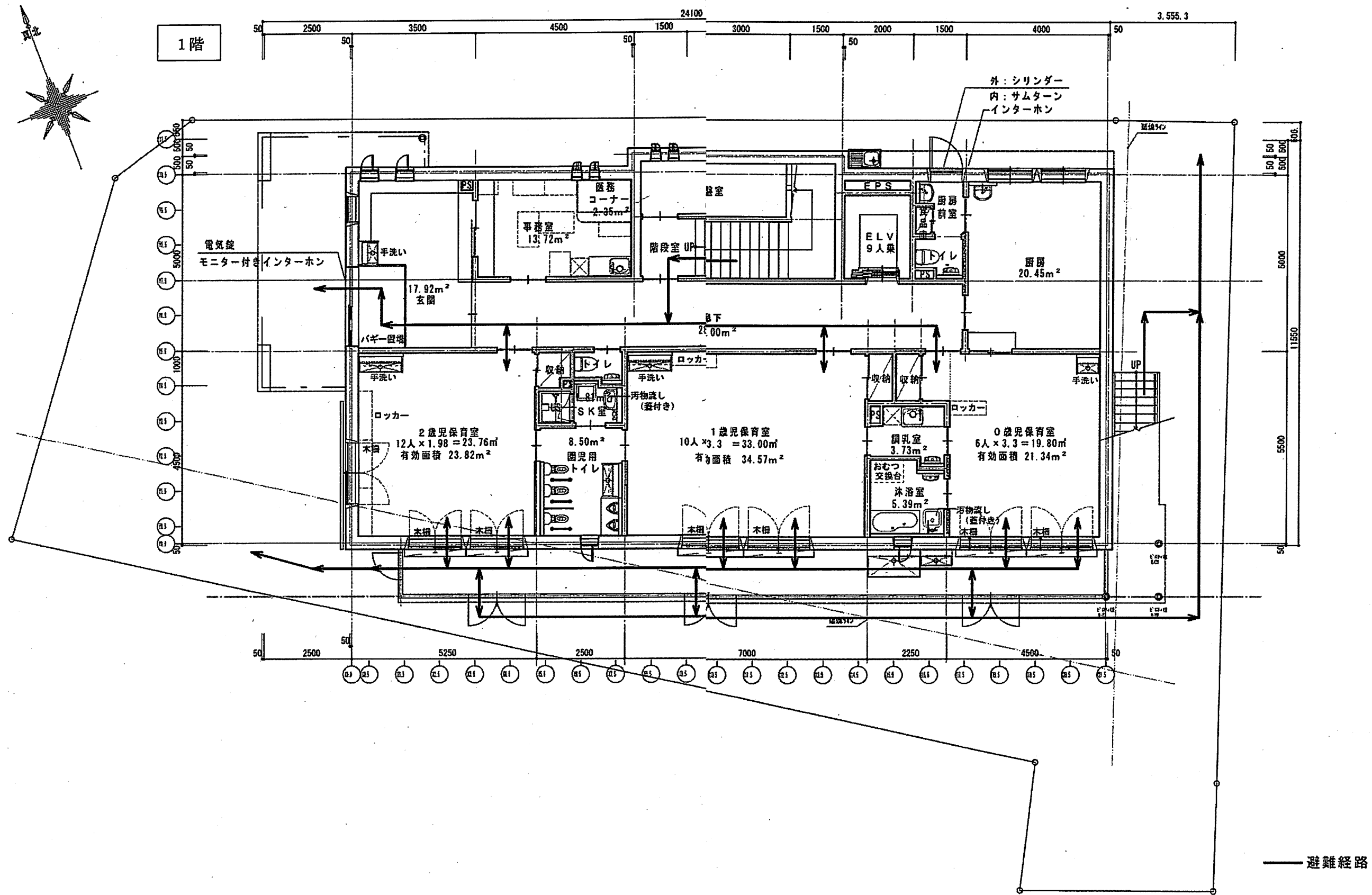
(仮称) にじいろ保育園東が丘・平面図
