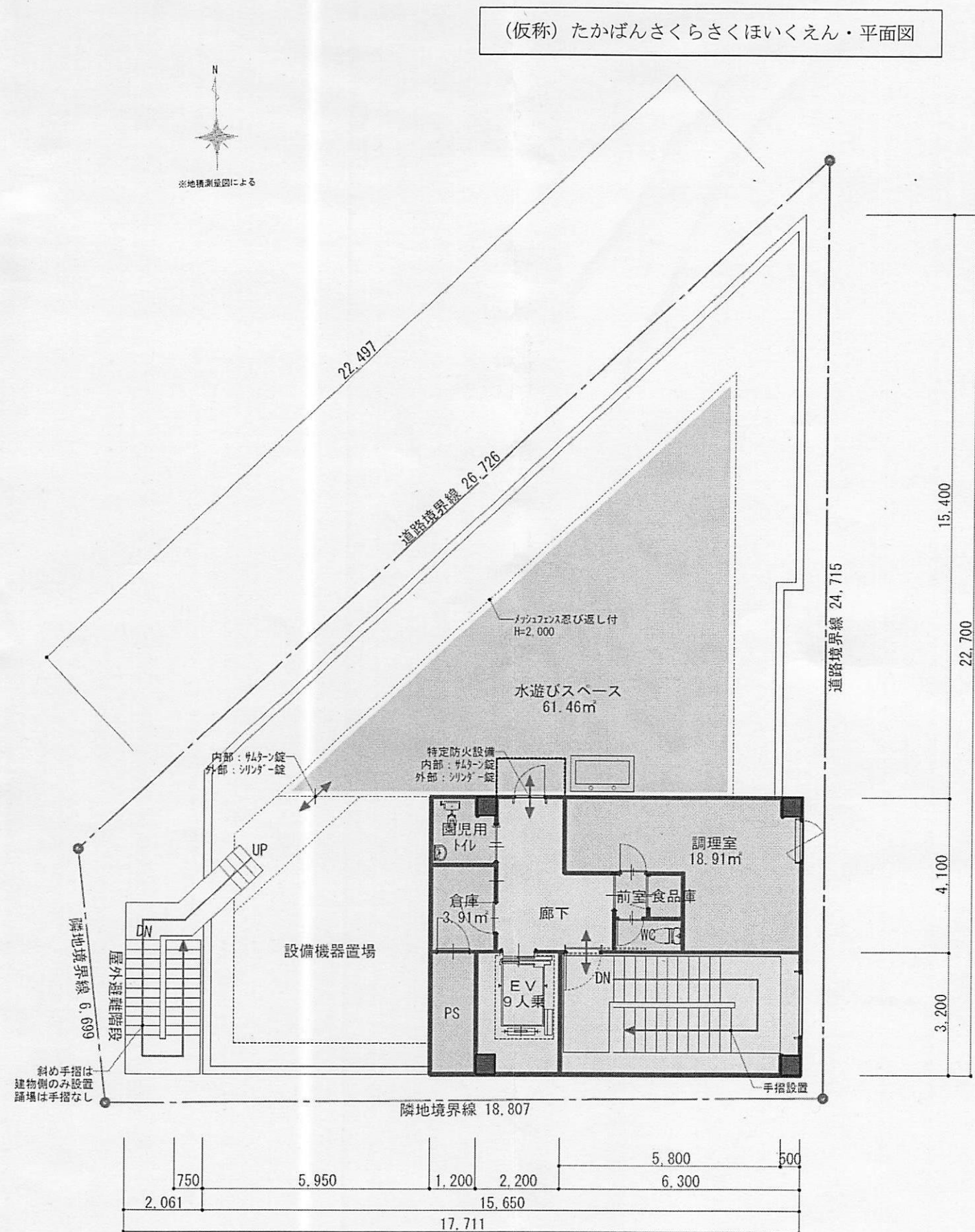
[ 4 階平面図 ]
