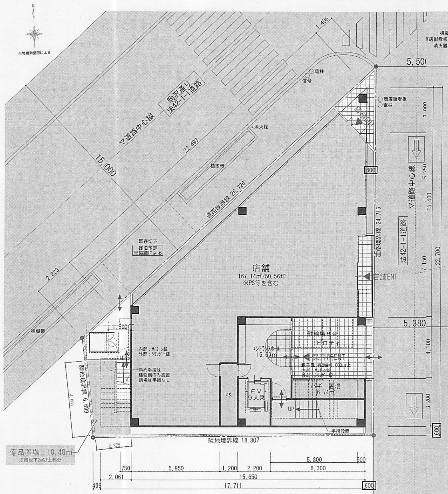
〔1階平面図〕
