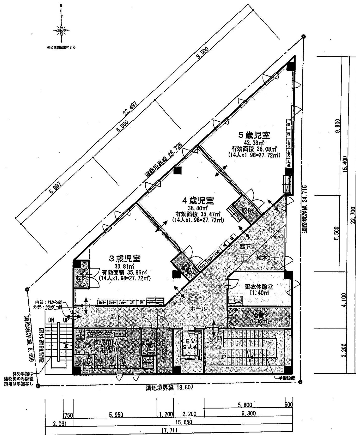
[ 3 階平面図 ]
