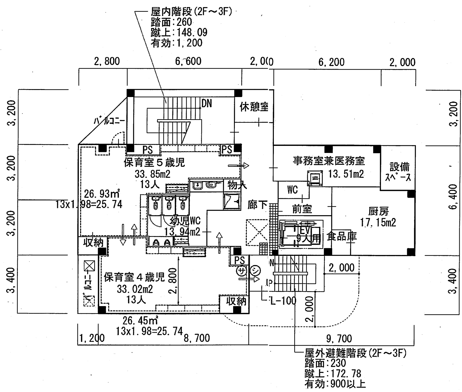
【3階平面図】
